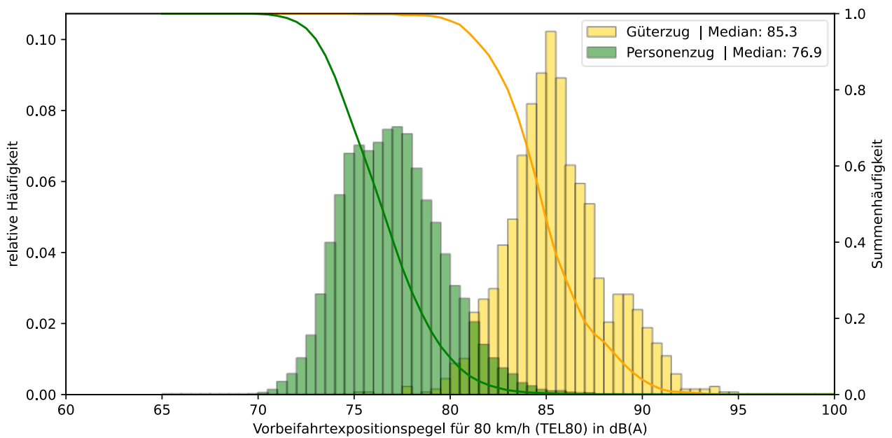
Abbildung 9. Relative Häufigkeitsverteilung und Summenhäufigkeit aller im Jahre 2025 gemessenen Vorbeifahrtexpositionspegel ( d = 7,5 \text{ m} ) für die Bezugsgeschwindigkeit 80 \text{ km/h} , getrennt nach Güter- und Personenzügen.
